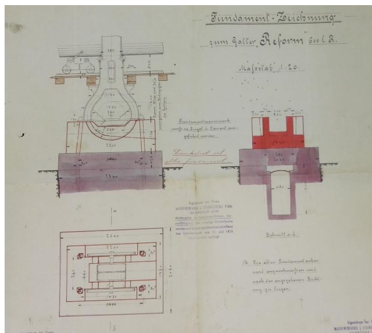
Část dokumentace rámové pily „Reform“ 600 mm od firmy Gebrüder Lein Pirna
