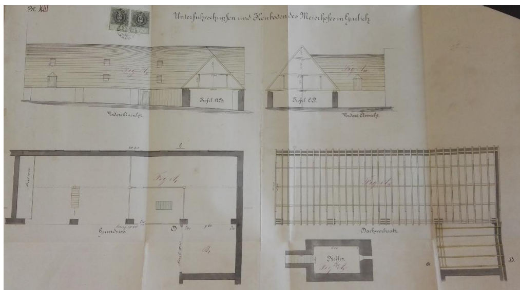
Stodola pro uskladnění zemědělského nářadí (H)
