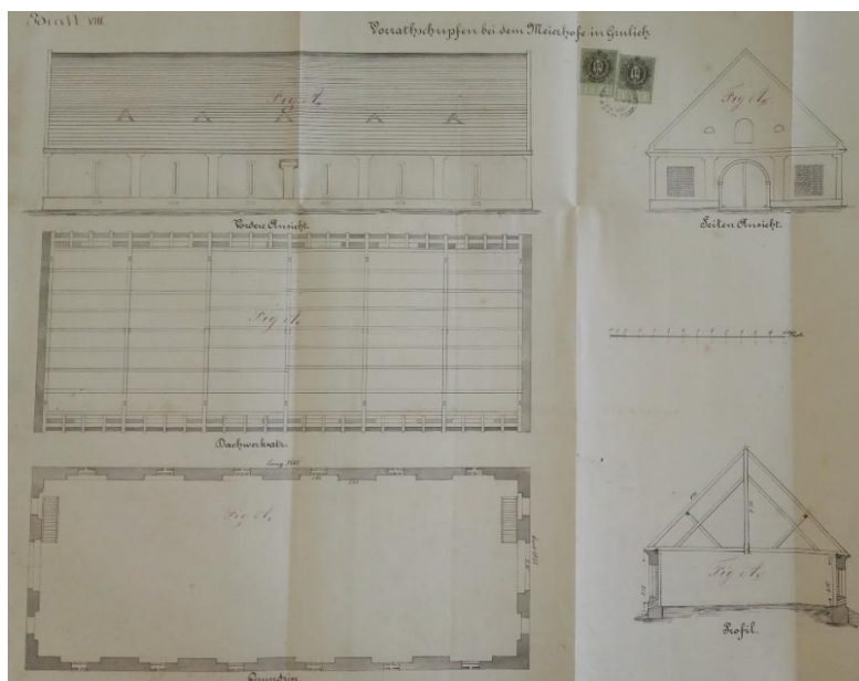
Sklad zásob v bývalé skladištní části
