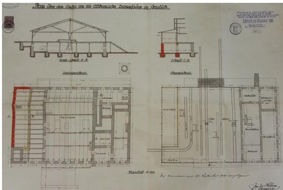
Výkresová dokumentace budovy pily
