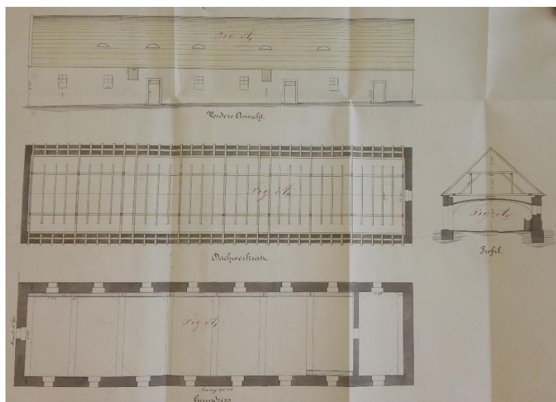
Chlén na skot (C), vpravo prostor klenuté řezárny, vlevo stání pro 58 kusů dobytka
