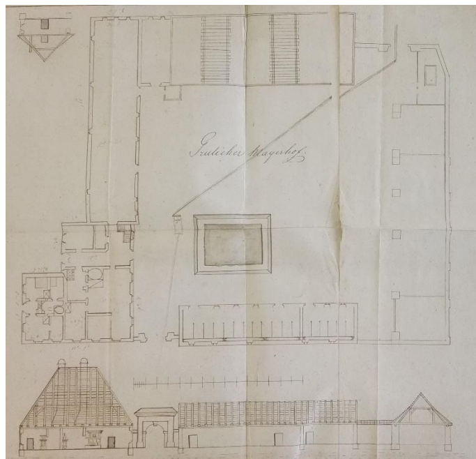
Celkový pohled na hospodářský dvůr centrály ( staré vyobrazení ještě před výstavbou sýpky)
