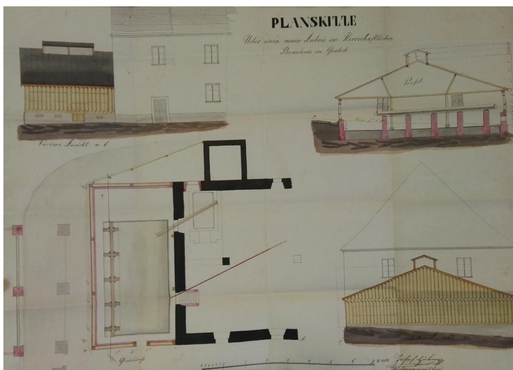
Zajímavý výkres zřejmě asi nikdy nerealizované přístavby budovy pivovaru. Zamýšlená přístavba se měla nacházet na západní straně budovy-při pohledu na půdorys vidíme úplně vlevo plot důchodního úřadu, cestu, vlastní přístavbu ( zřejmě asi další sladovny?). Vpravo nahoře pak čtvercový prostor (základy vstupu do ředitelství)
