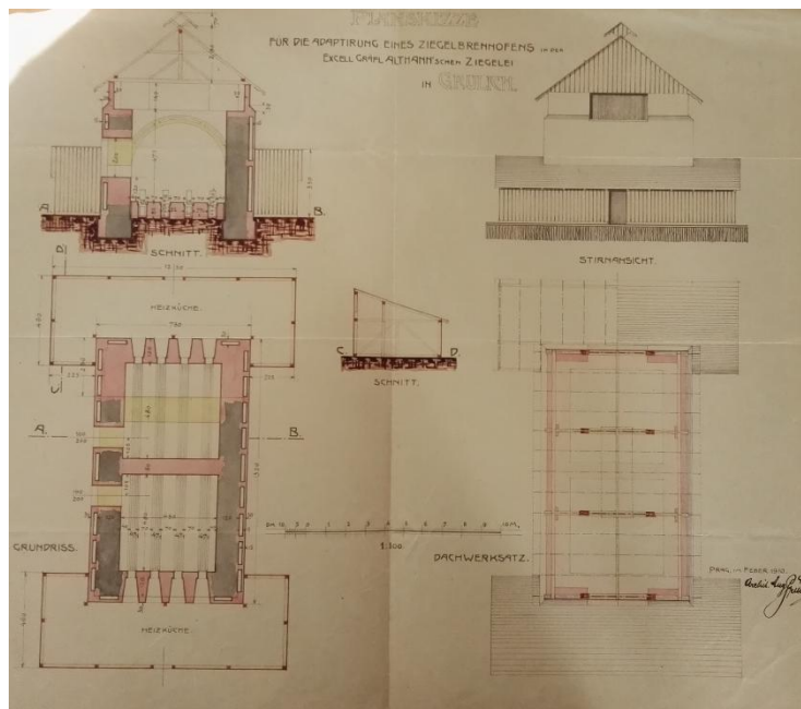
Nová cihlářská pec (F)
