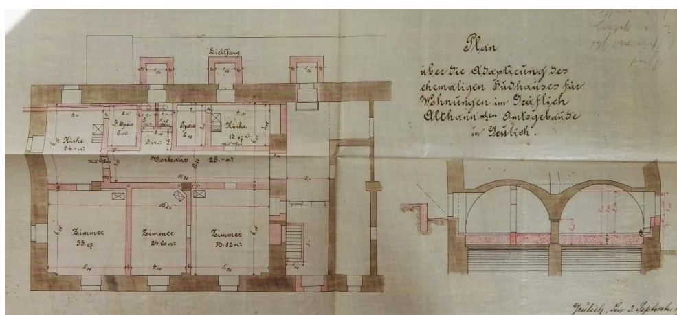
Přestavba západních prostor pivovaru na dva byty. Byty měly dělenou dispozici. Z pokojů se do kuchyní a na záchod muselo přes společnou chodbu. Všimněme si že kvůli získání světla se musely v severní zahloubené stěně udělat šachty pro okna.
